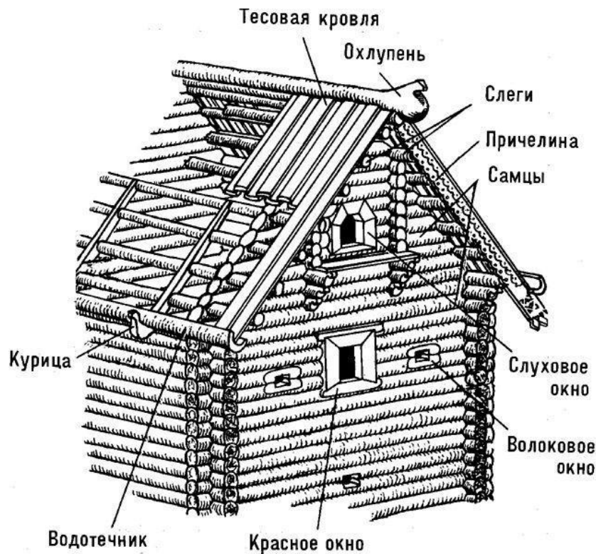
Рис. 1. Схема устройства самцовой кровли
