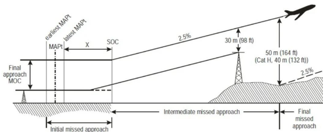
Рис. 1. Схема повторного захода на посадку
