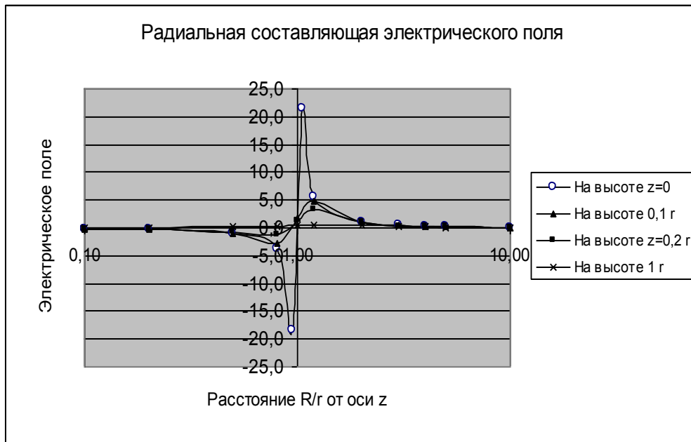
Рис. 9. Радиальная составляющая электрического поля кольца
