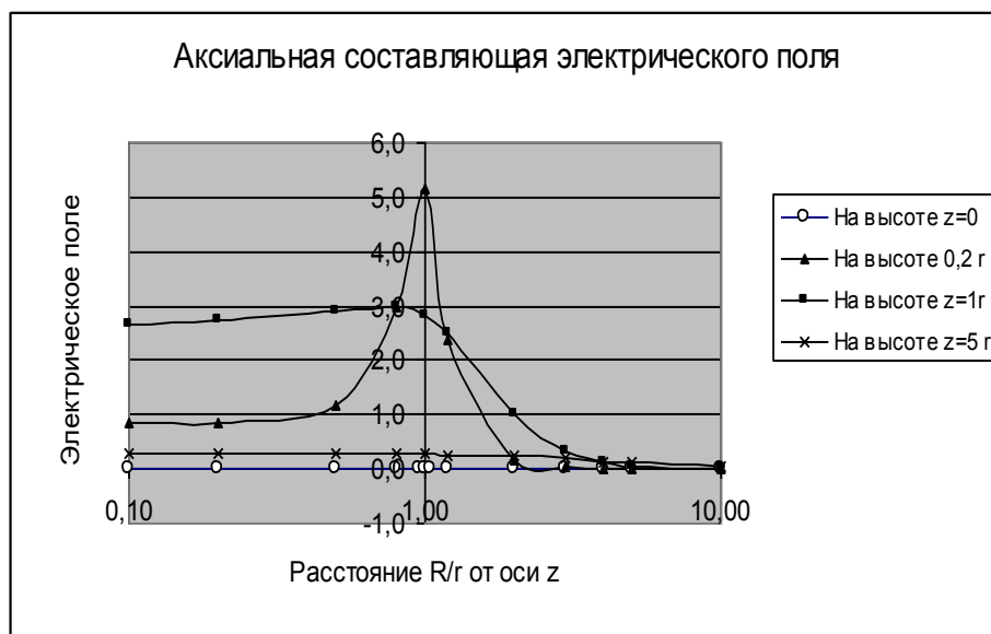
Рис. 10. Аксиальная составляющая электрического поля кольца
