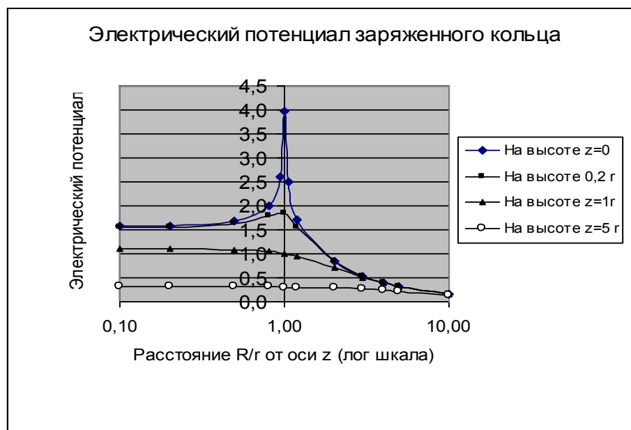
Рис. 8. Графики распределения потенциала кольца в пространстве
