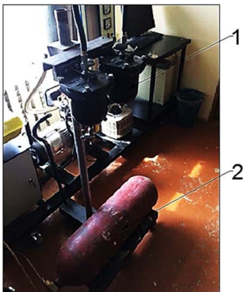
Рис. 3.10. Установка очистки биогаза: 1 – разработанный фильтр, 2 – метановый баллон
